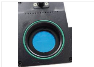
hintere Schutzlinse, Größe 30 x 2 mm
