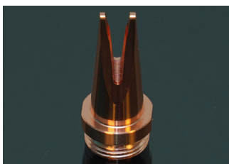
Schweißdüse H40-H
