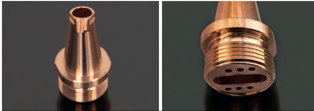
Schweißdüse AS-10
